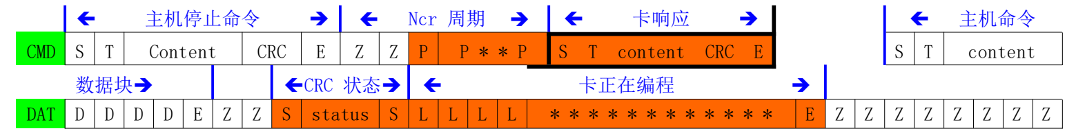
图 4-24：卡传输 CRC 状态期间停止传输
