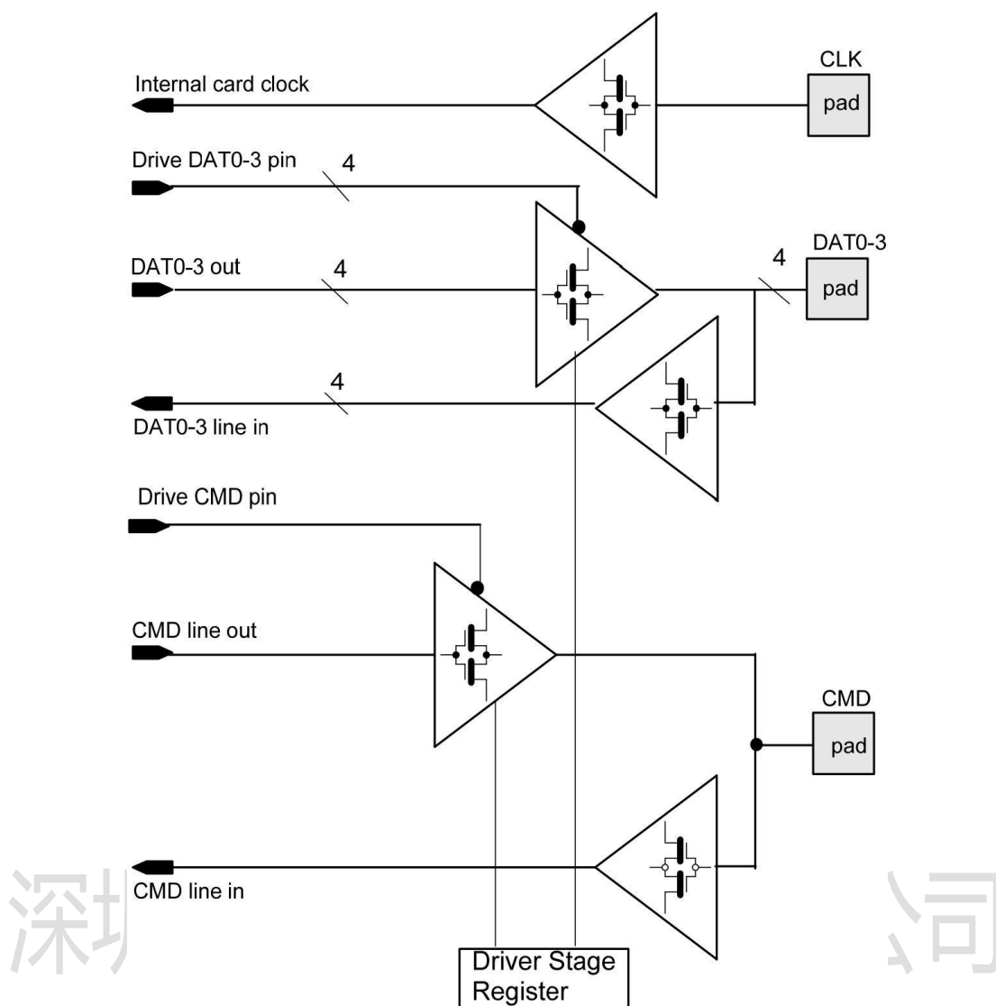
图 6-5 SD 卡总线驱动
