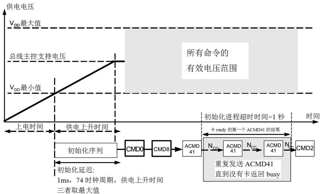
图 6-4 上电流程
