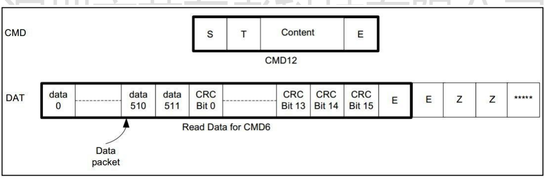
图 4-7 CMD6 期间发送 CMD12 Case 2
