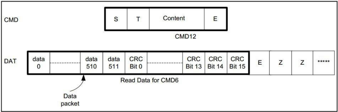
图 4-6 CMD6 期间发送 CMD12 Case 1
