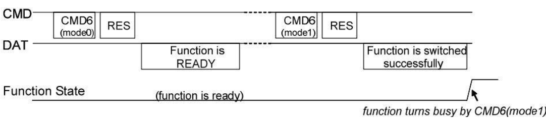
图 4-8 切换功能流程实例
