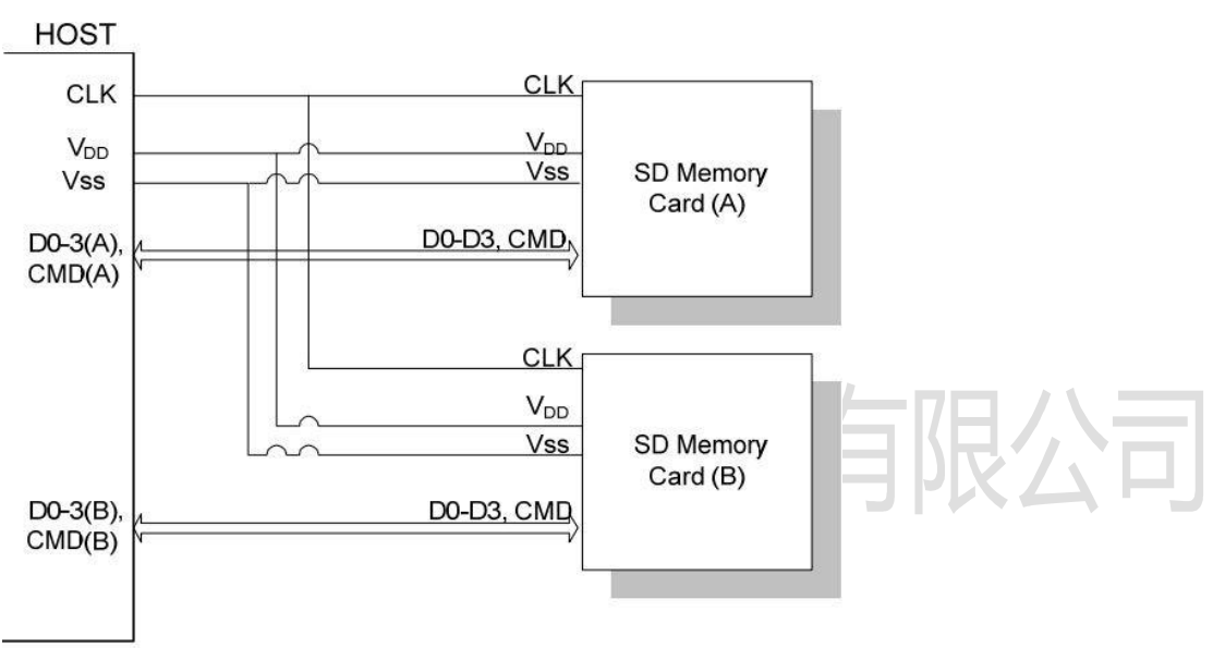
图 3-2 SD 卡总线拓扑
