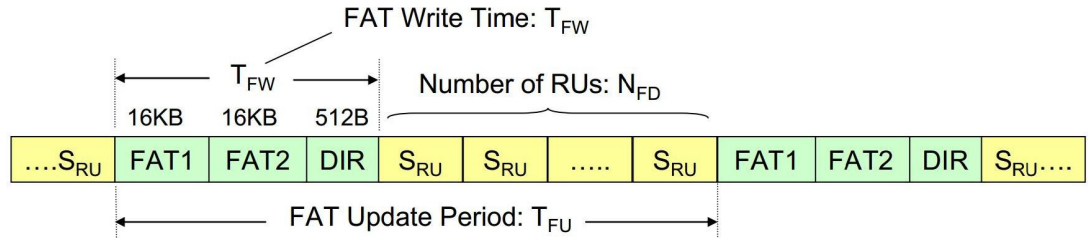
图 4-31 典型 FAT 更新序列
