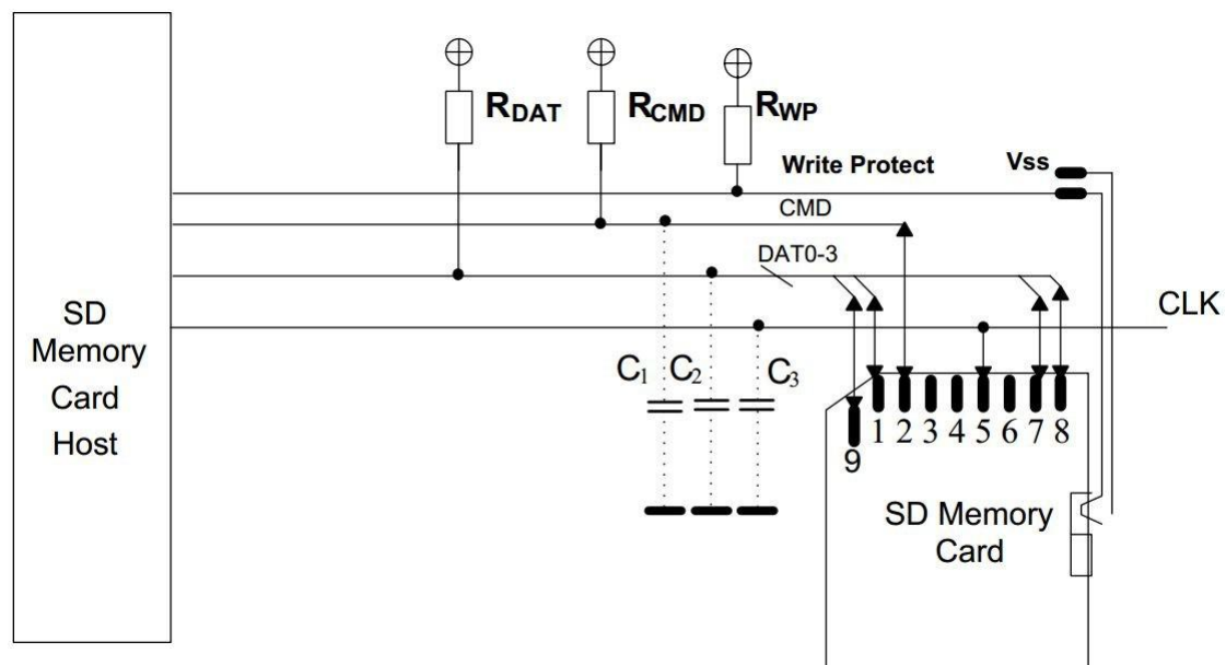
图 6-1 总线电路图
